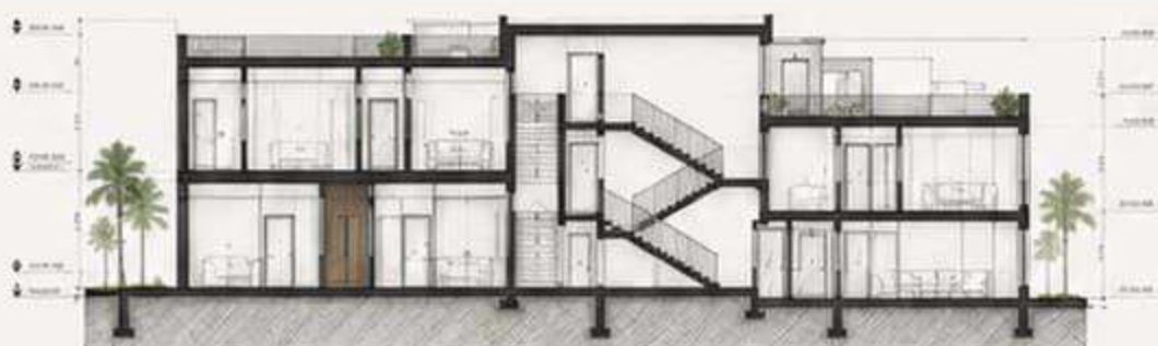
قطاع رأسي A-A
