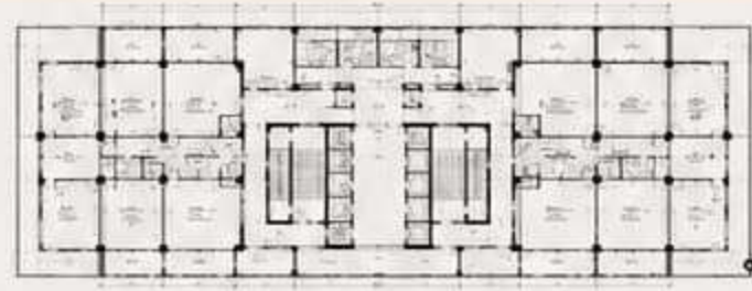
مخطط الدور النموذجي (إداري)
